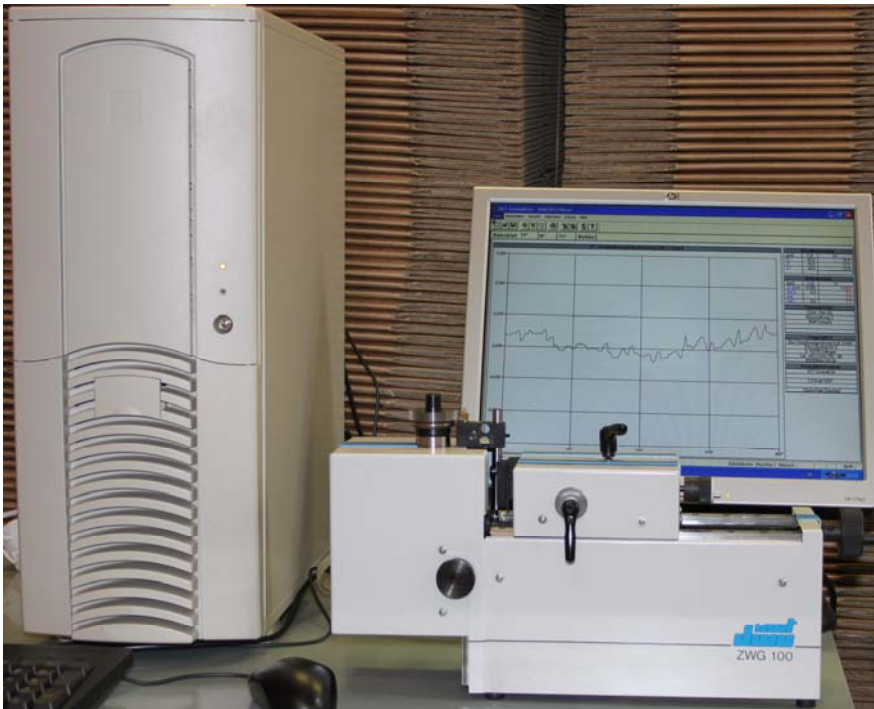
ZWG100N für Kleinverzahnung
