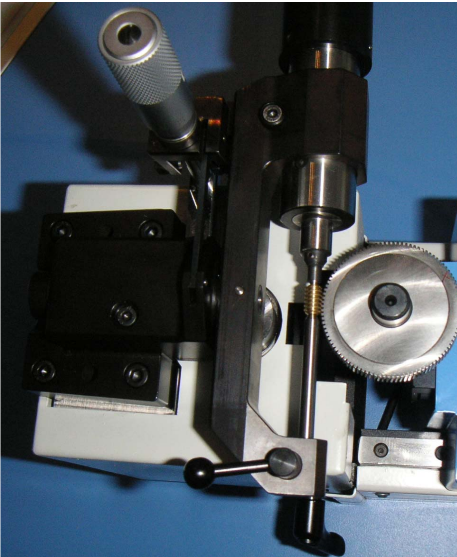
ZWG100 mit Schneckenaufsatz
