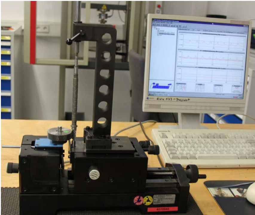
ZWG100H mit langem Widerlager für Ritzel-Motorwellen
